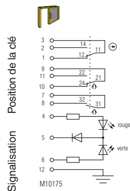
Fig. 2 : Verrouillage à l'état désactivé: clé retirée
