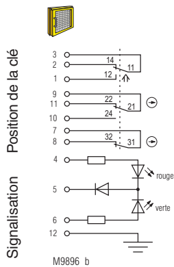
Fig. 1 : Verrouillage à l'état activé: clé insérée
