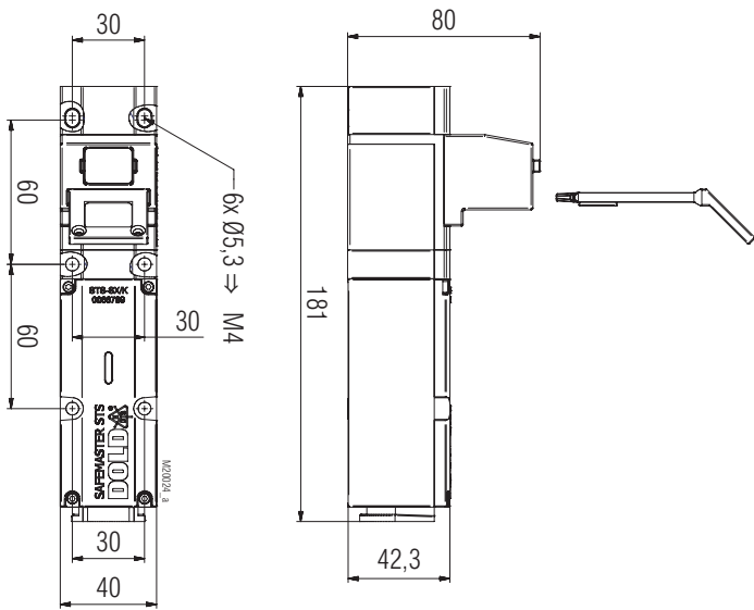
SX01M/K Tolérances générales \pm 2\%
