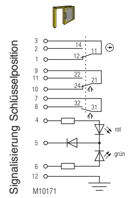
Bild 2: Verriegelung im deaktivierten Zustand: Schlüssel entnommen
