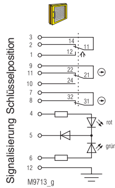
Bild 1: Verriegelung im aktivierten Zustand: Schlüssel gesteckt
