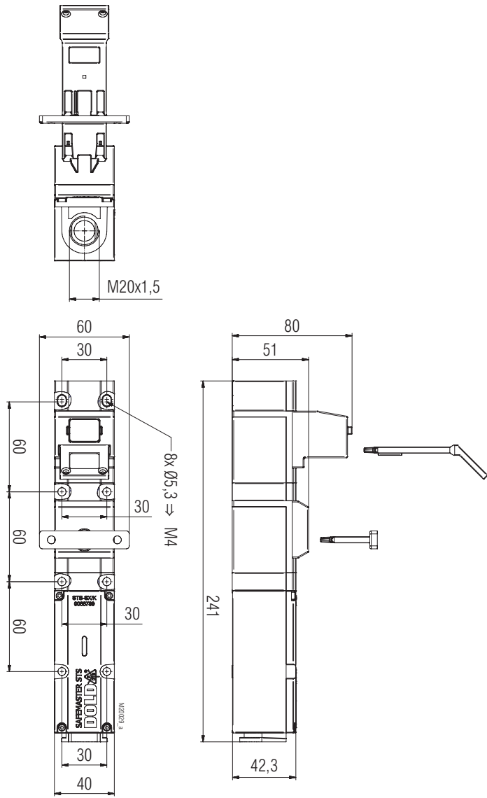
SXB01M/K Tolérances générales ± 2%
