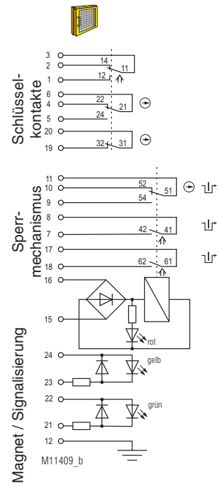
Bild 2: Zuhaltung im deaktivierten Zustand: Magnet entriegelt, Schlüssel entnommen
