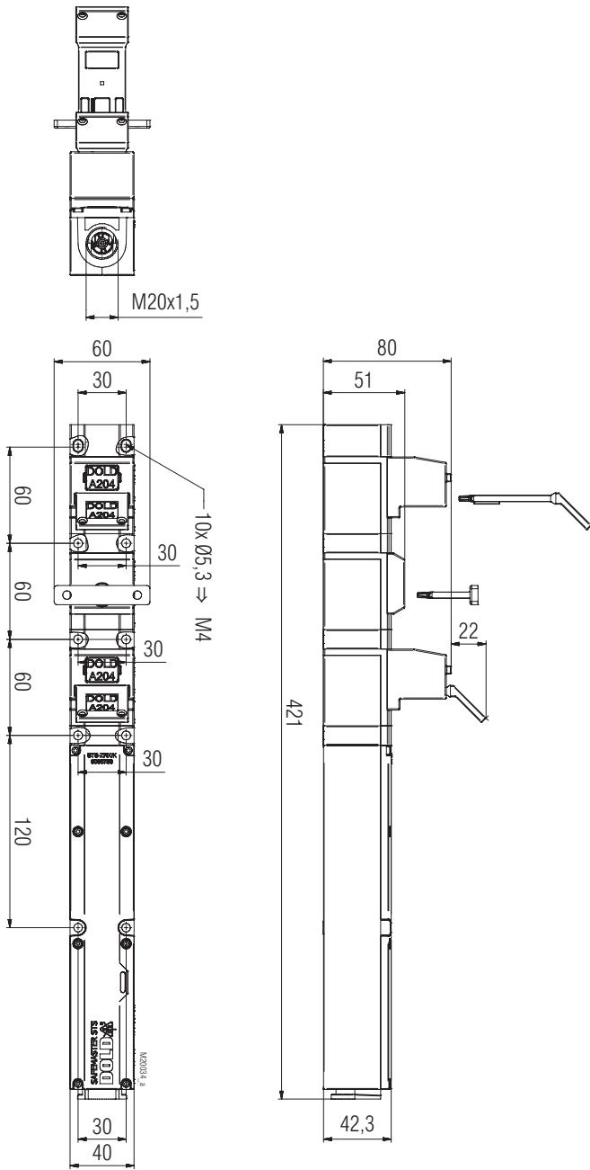
YRX10B01M/K Freimaßtoleranzen ± 2%
