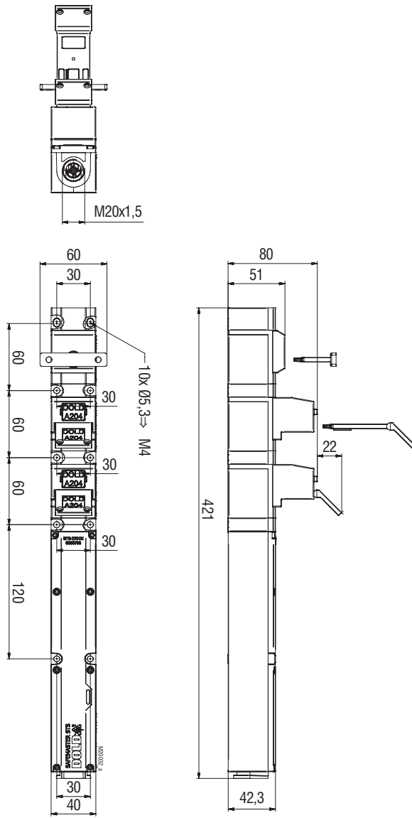
YRX11BM/K Freimaßtoleranzen ± 2%
