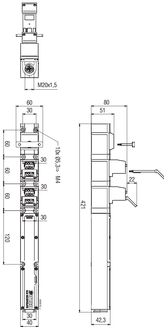
YRX11BM/K Tolérances générales ± 2%
