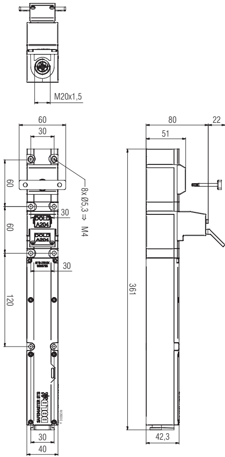
YRX10BM/K Freimaßtoleranzen ± 2%
