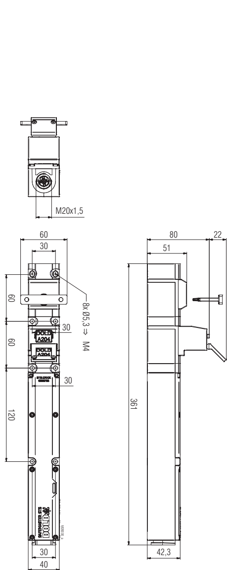
YRX10BM/K Tolérances générales ± 2%
