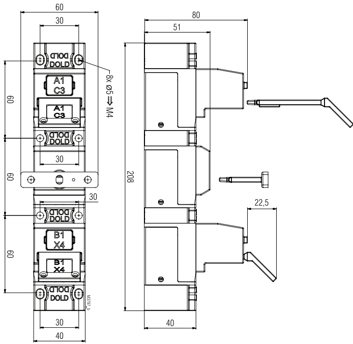
Illustration: M10B01M Tolérances générales \pm 2\%
