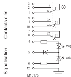
Fig. 2 : Verrouillage à l'état désactivé: clé insérée, actionneur retiré, porte ouverte
