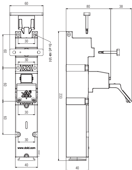
RX10A Tolérances générales ± 2%
