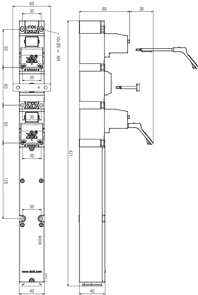
YRH10B01M Tolérances générales ± 2%
