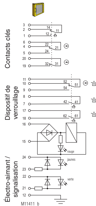
Fig. 2 : Gâche à l'état désactivé : Électro-aimant déverrouillé, 1 re Clé à retirer, 2 e Clé insérée
