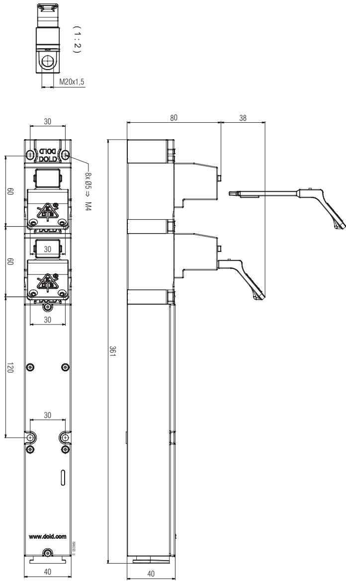
Abbildung: YRX11M Freimaßtoleranzen \pm 2\%
