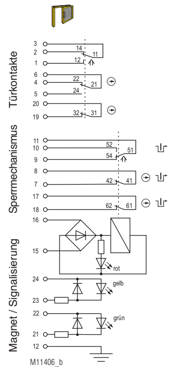
Bild 2: Schalter im aktivierten Zustand: - YRXKM: Sperrmechanismus verriegelt, Betätiger entnommen - YRXK01M: Schlüssel gesteckt, Betätiger entnommen, Sperrmechanismus aktiviert
