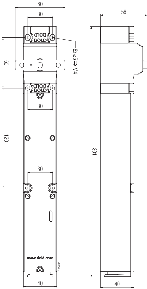
YRXXKM Tolérances générales ± 2%
