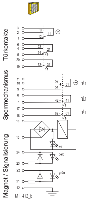
Bild 1: - YRXKM: Schalter im aktiven Zustand, Betätiger gesteckt, Sperrmechanismus entsperrt - YRXK01M: Zuhaltung im aktivierten Zustand, Betätiger gesteckt, Sperrmechanismus entsperrt
