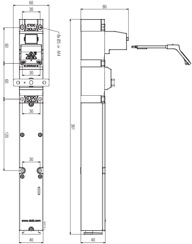
YRXXK01M Tolérances générales ± 2%
