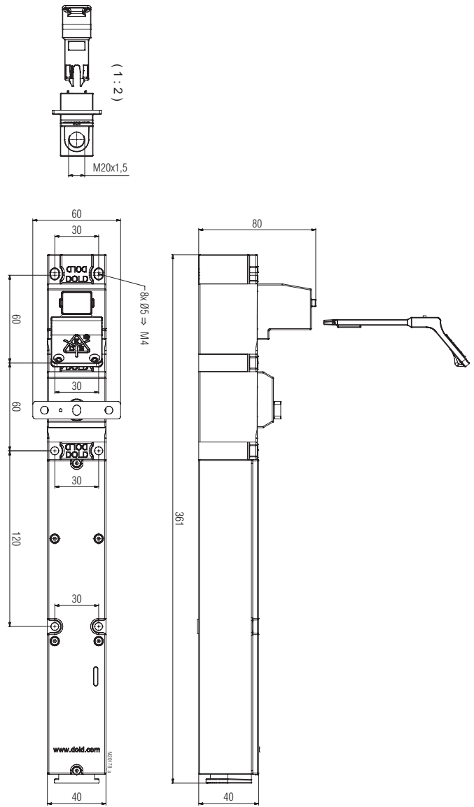
Abbildung: YRXK01M Freimaßtoleranzen \pm 2\%
