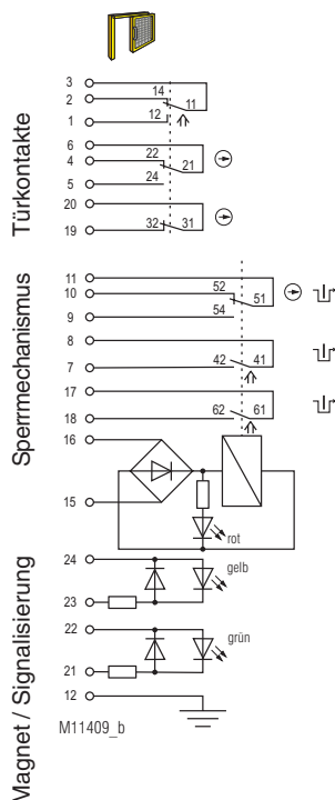
Bild 3: Schalter im deaktivierten Zustand: - YRXKM: Sperrmechanismus entriegelt, Betätiger entnommen - YRXK01M: Zuhaltung im deaktivierten Zustand, Schlüssel gesteckt, Sperrmechanismus entriegelt, Betätiger entnommen
