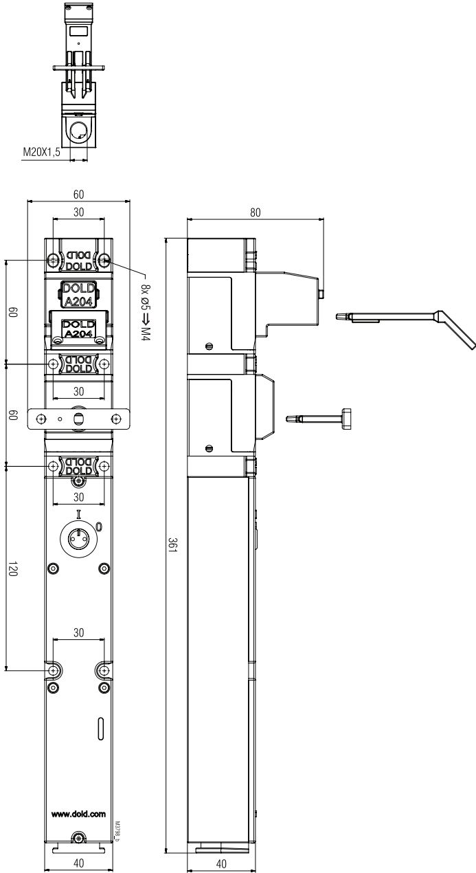
ZRHB01M Tolérances générales \pm 2\%
