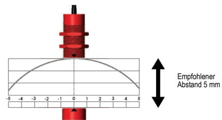
Abb. 3: Aktivierungsbereich Serie ZCode bei 5 mm Nennabstand
