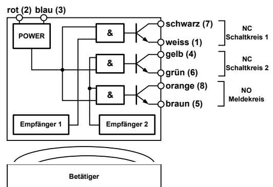
Abb. 2: Blockschaltbild
